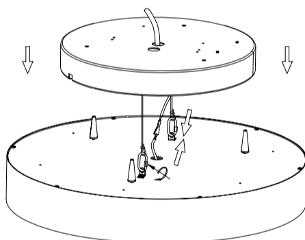
Väggmontering
